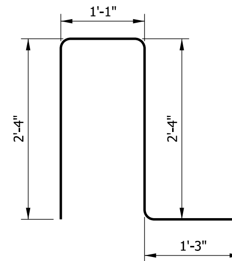
4700E x 7'-0"
