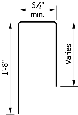
#4 BENT BAR
