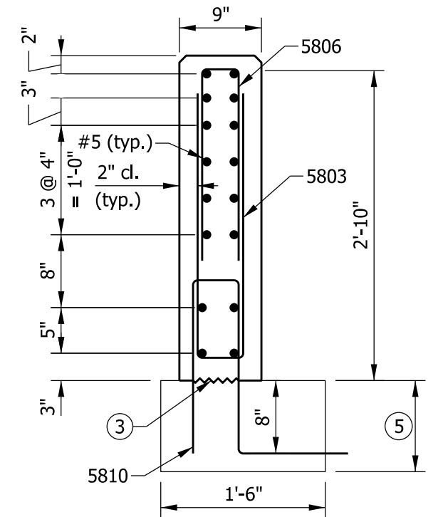
SECTION D-D
